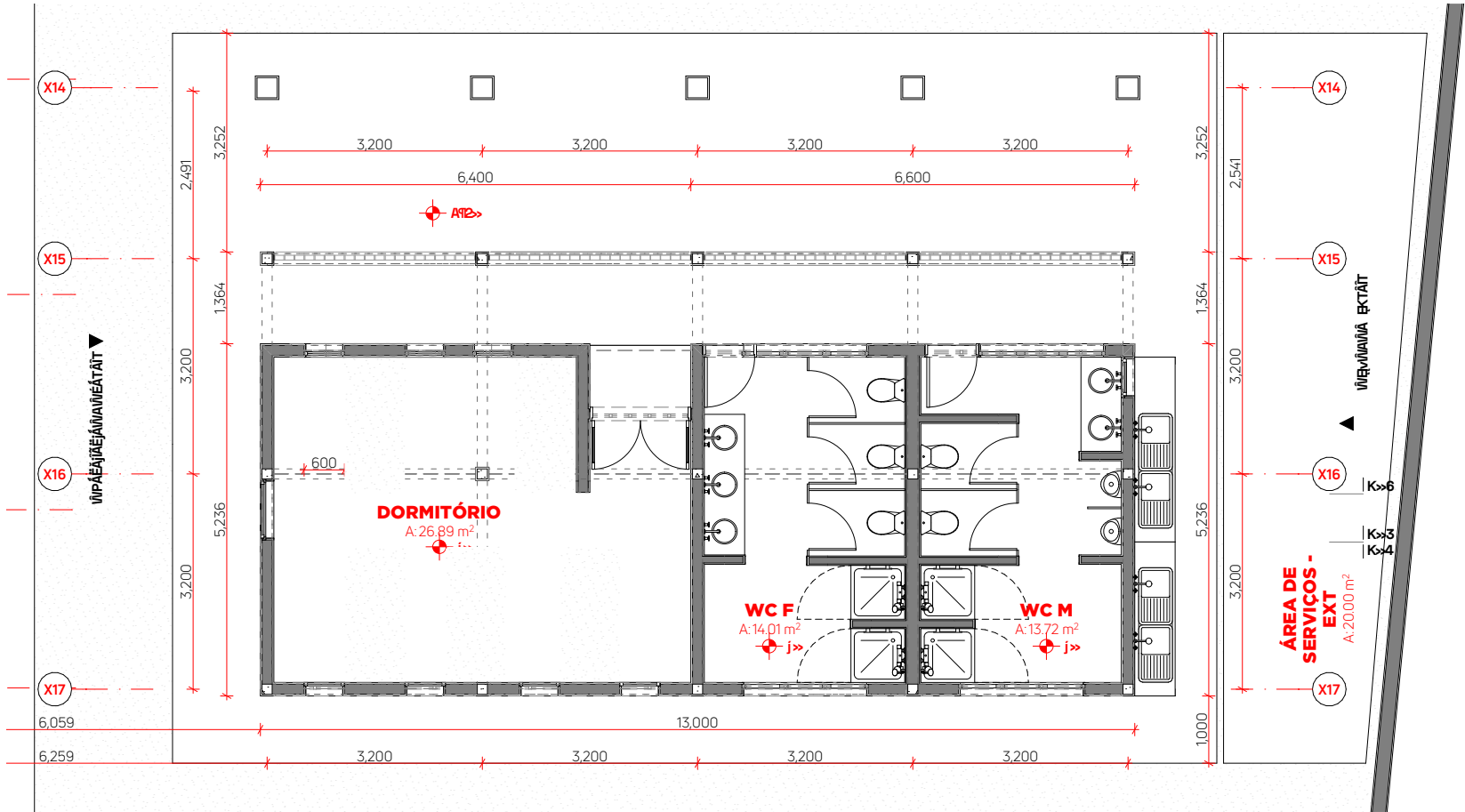
Panta de piso Cotado - Dormitório
