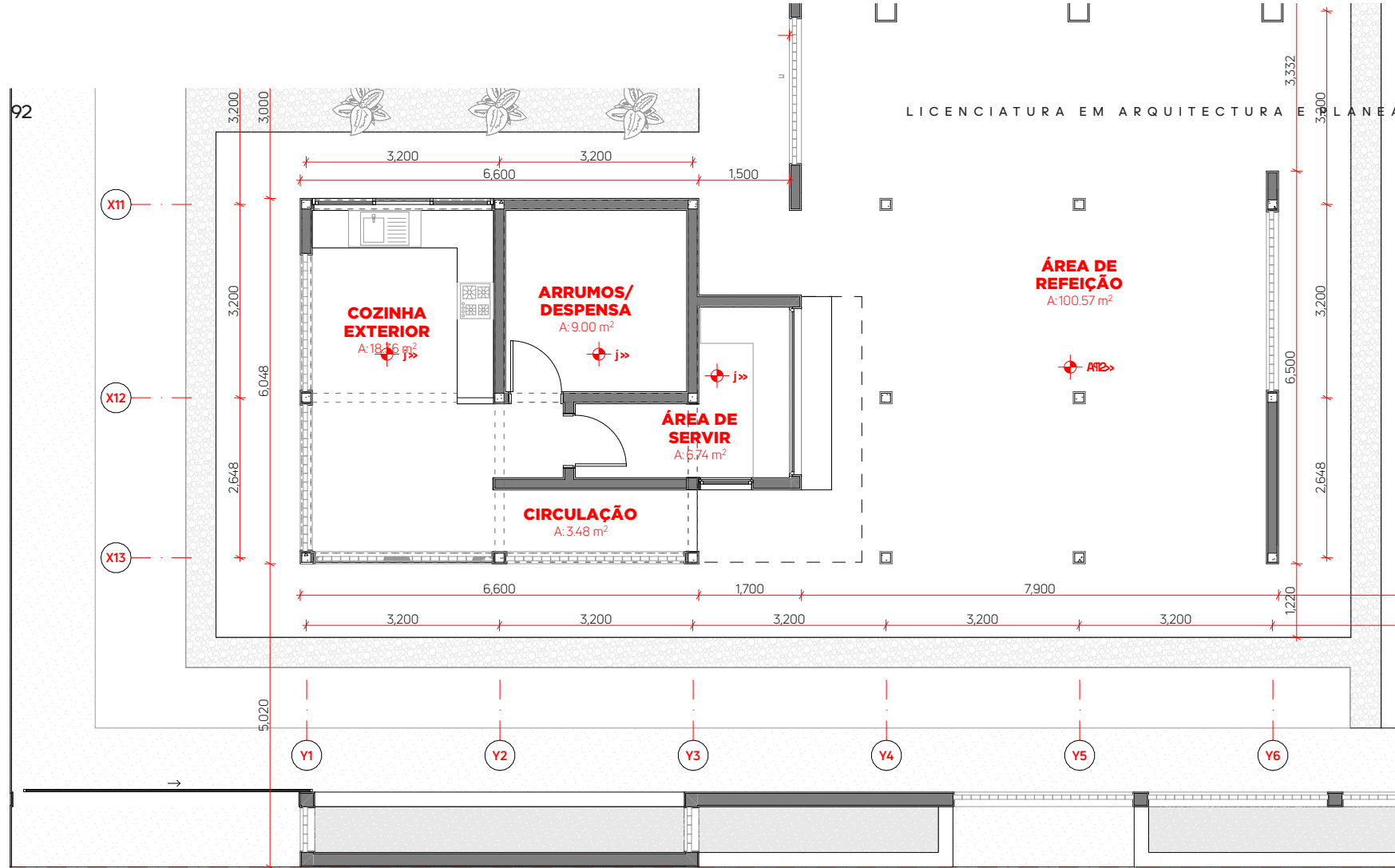
Planta De piso Cotado – Administração
