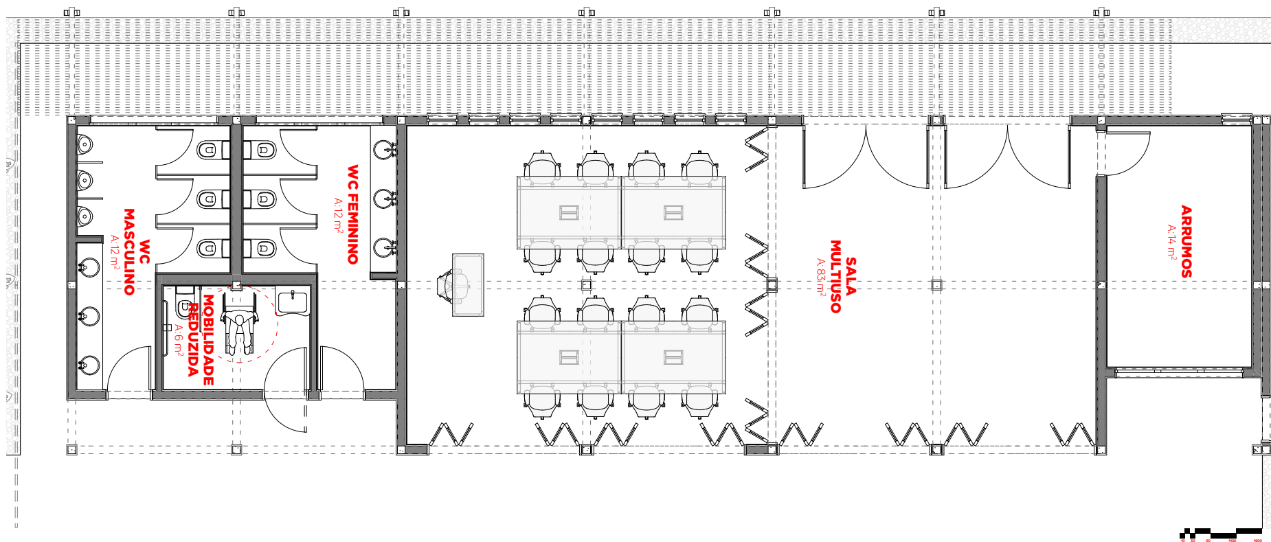
Planta de piso Mobilado - Sala de Aulas ESC1/100
