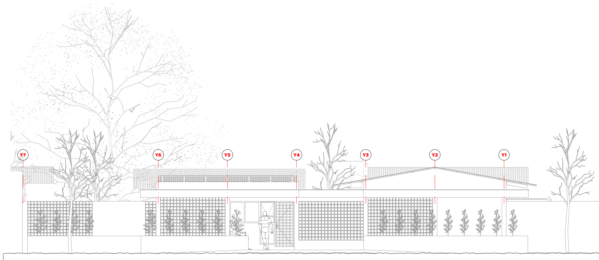
Alçado Geral - Norte ESC 1/100
