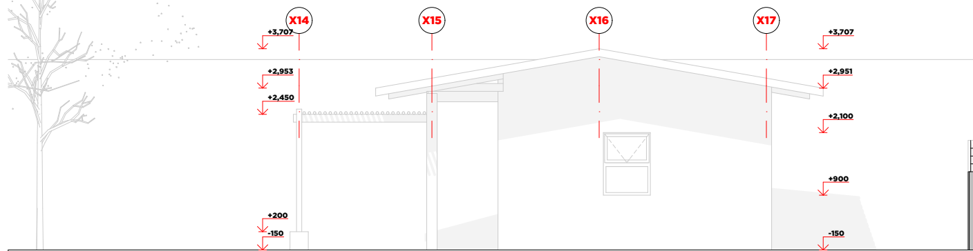
Alçado Poente - Dormitório ESC 1/100
