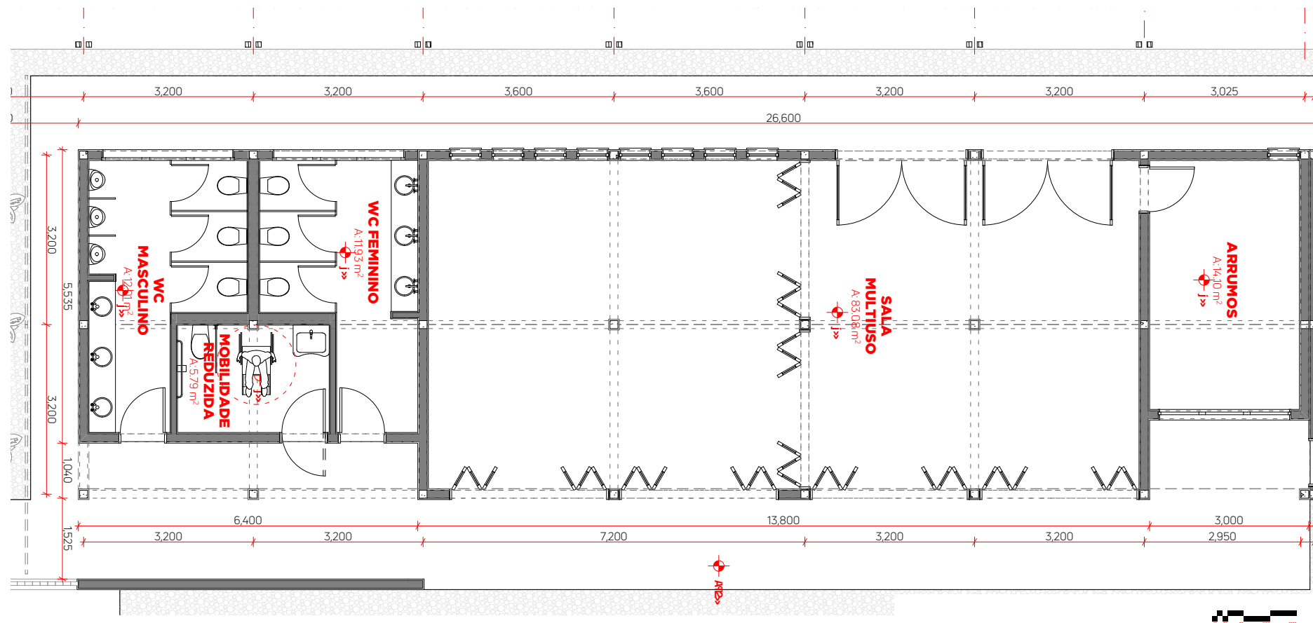
Planta de piso Cotado- Sala de Aulas
