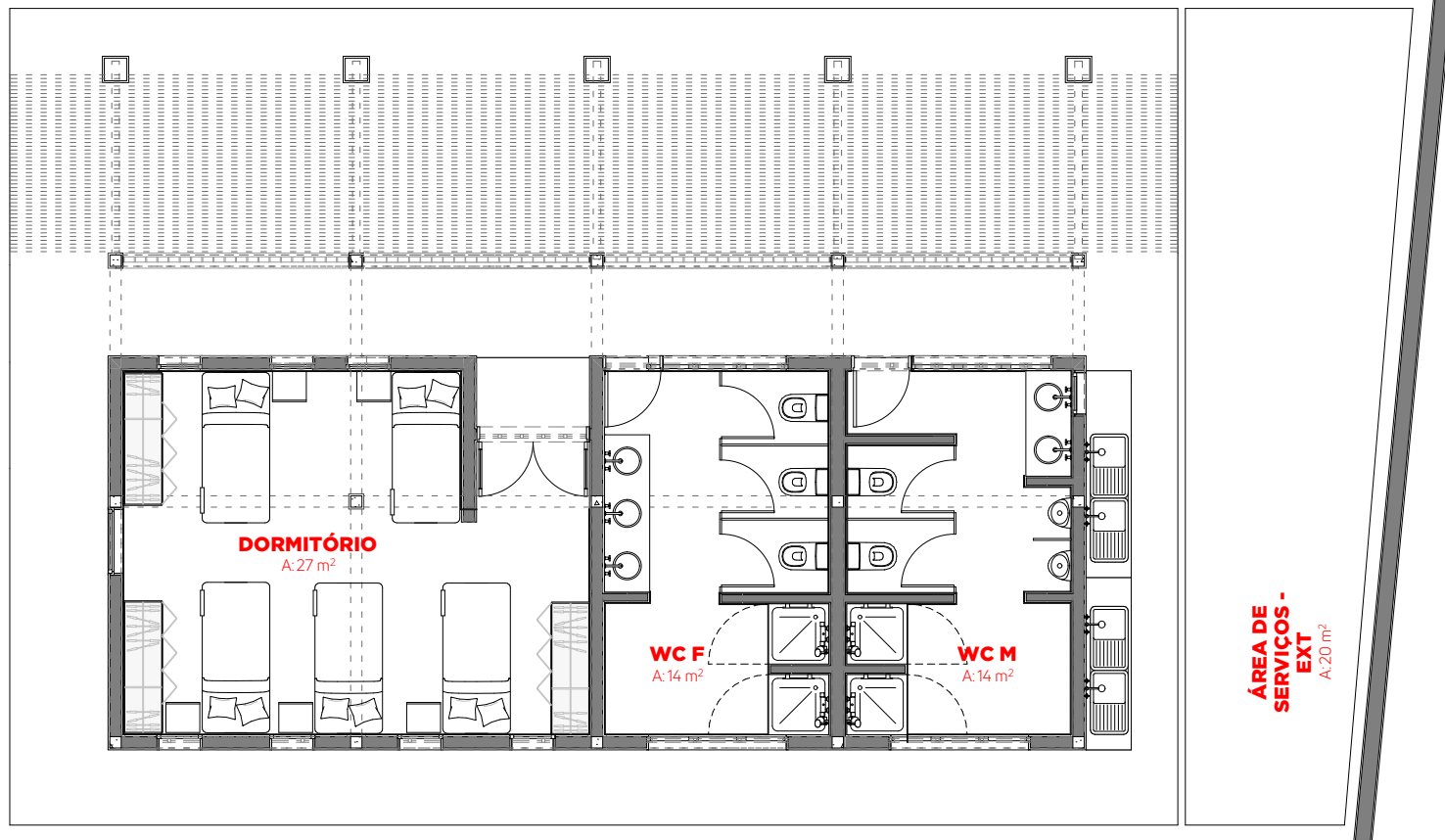
Panta de piso Mobilado – Dormitório ESC 1/100
