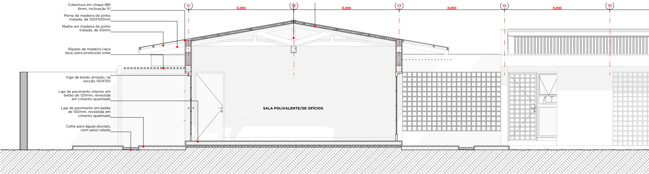
Corte - Sala de Aulas
