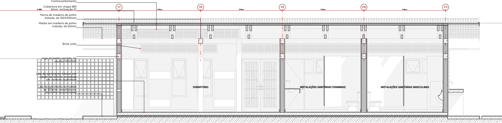
Corte - Dormitório ESC 1/50
