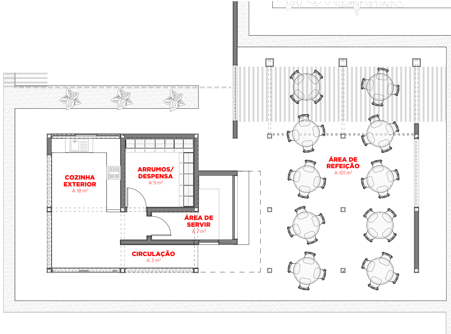
Planta De piso Mobilado - Cozinha e Refeitório
