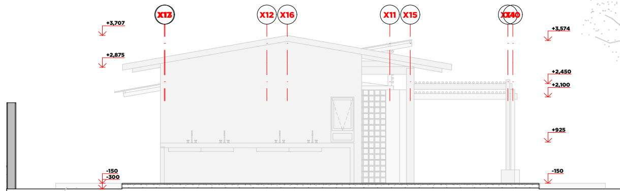
Alçado Poente - Dormitório ESC 1/100
